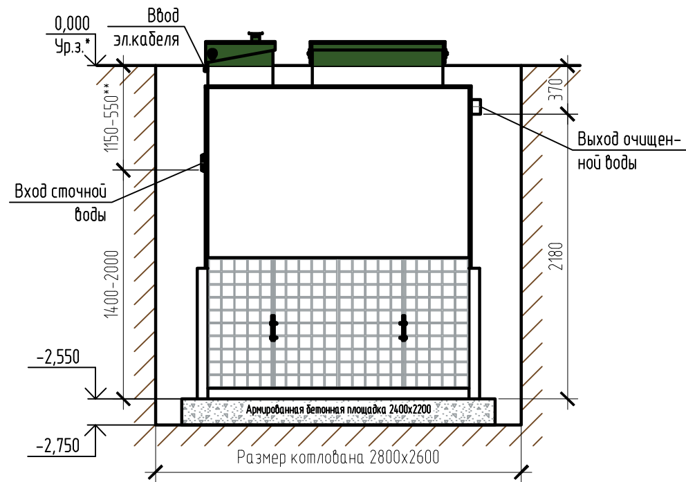
Вид А
