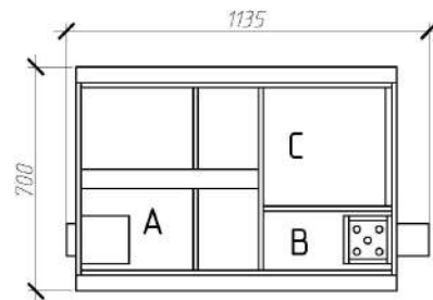
Габаритные размеры ОТП-1
