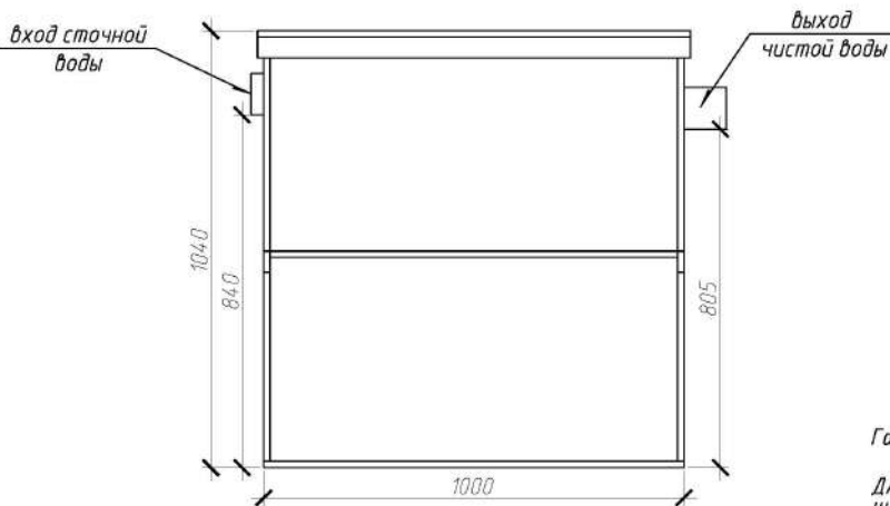
Вид сбоку
